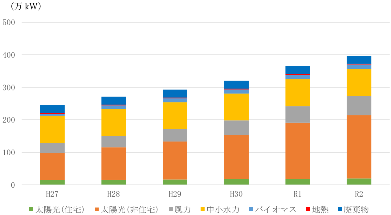
図 3-4 北海道における新エネルギー導入実績 (設備容量)
