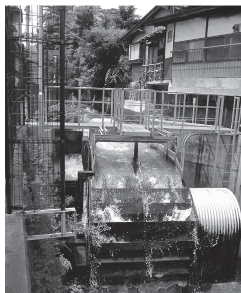
上掛け水車方式の元気くん2号
